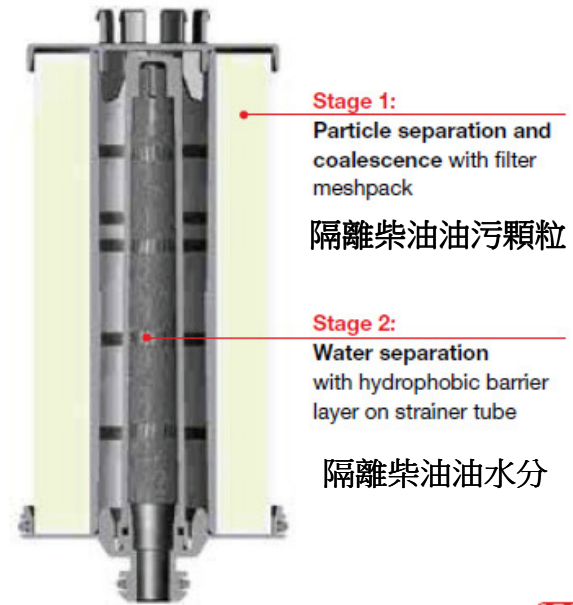
柴油濾芯結構剖視說明
